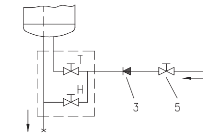
Otevřený (průtokový) systém
