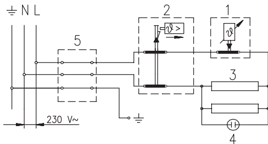
Schema električnog spajanja
