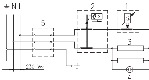
Шема електричног везивања
