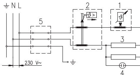
Электросхема
