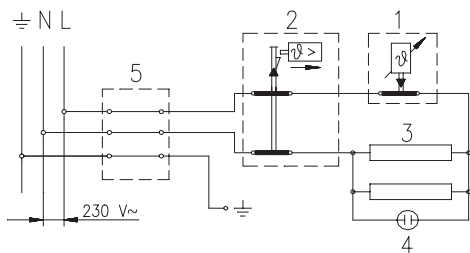
Elektrisk sh ma
