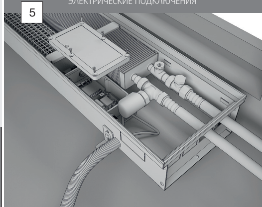
ЭЛЕКТРИЧЕСКИЕ ПОДКЛЮЧЕНИЯ
